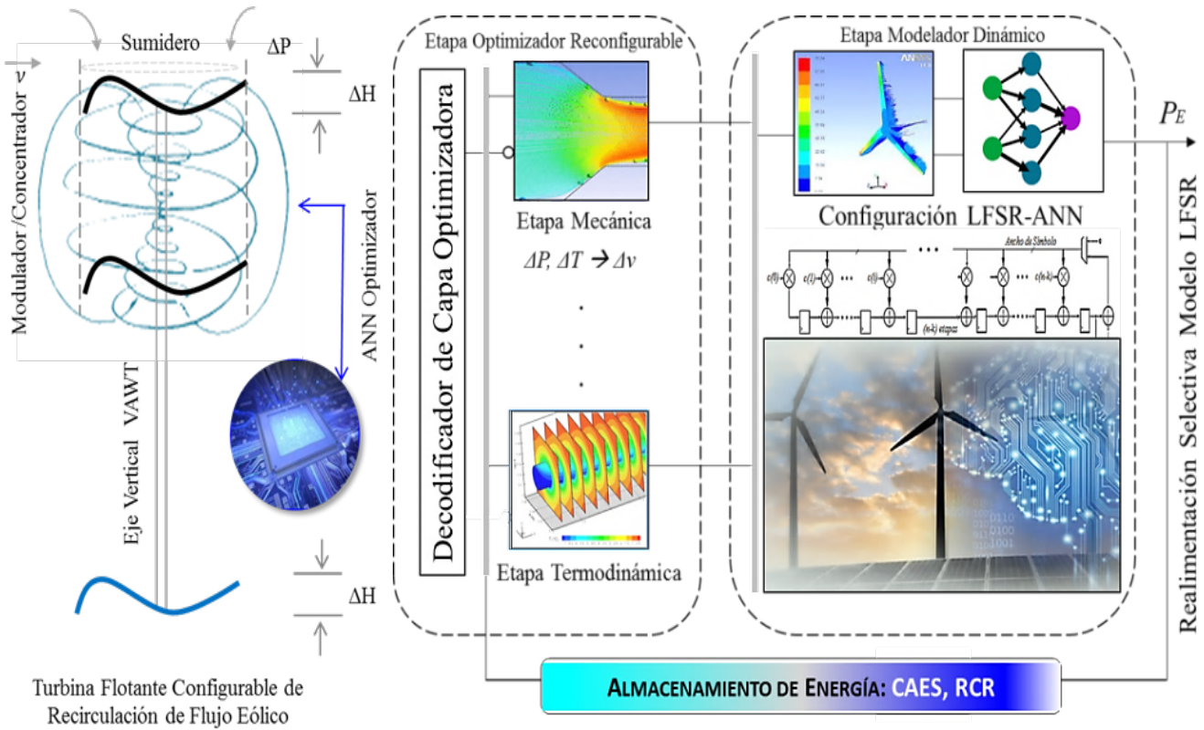
Figura 1. Esquema Conceptual de Eólica Reconfigurable
